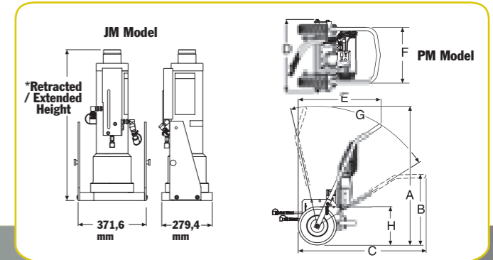
660 mm Jack Module
